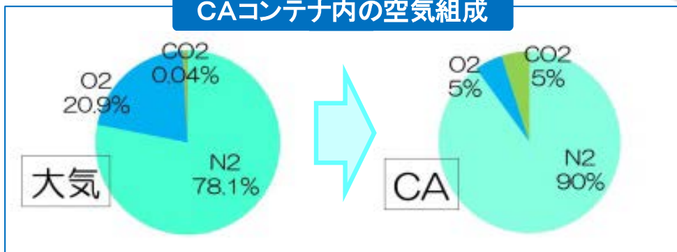
CAコンテナ内の空気組成
