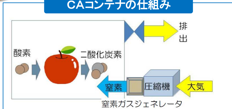
CAコンテナの仕組み
