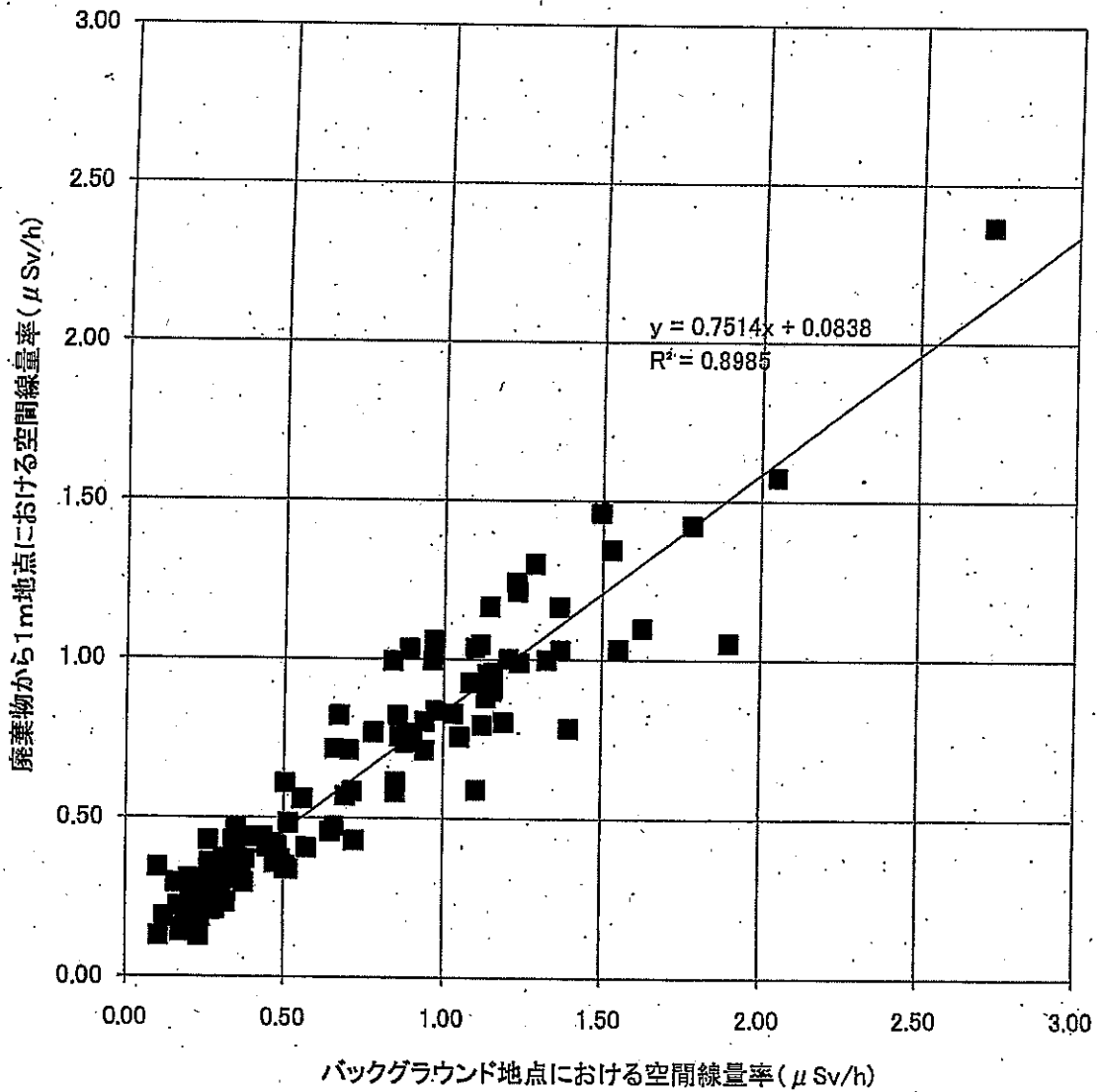
廃棄物から1m地点における空間線量率とバックグラウンド地点における空間線量率の関係(中央値)
